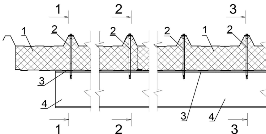
Рисунок 12. Сечение по прогону кровельных панелей крайнего и последующего рядов с указанием разрезов.
