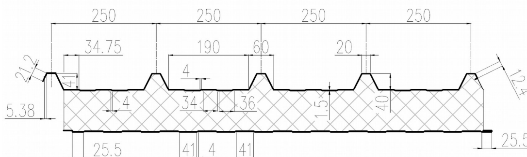
Рисунок 1. Геометрия кровельной сэндвич-панели
