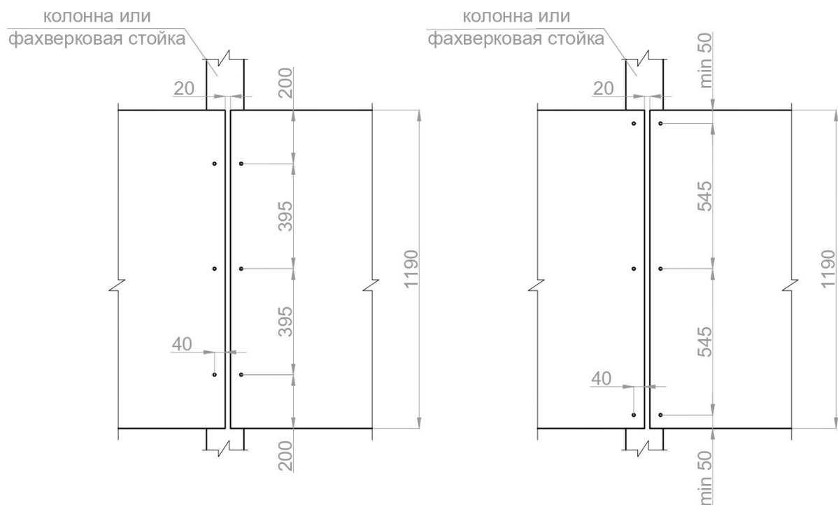
Рисунок 11. Стеновые панели ПСТ второго и последующих рядов. Варианты крепления к колонне или фахверку при горизонтальной раскладке.
