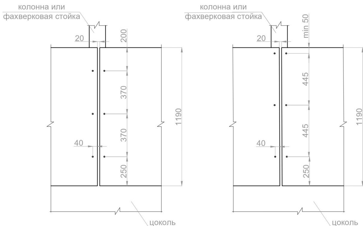
Рисунок 10. Стеновые панели ПСТ первого ряда. Варианты крепления к колонне или фахверку при горизонтальной раскладке.
