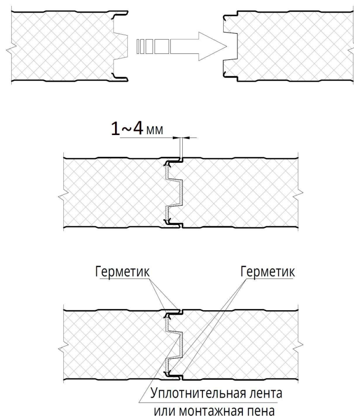
Рисунок 7. Замок стеновых панелей
