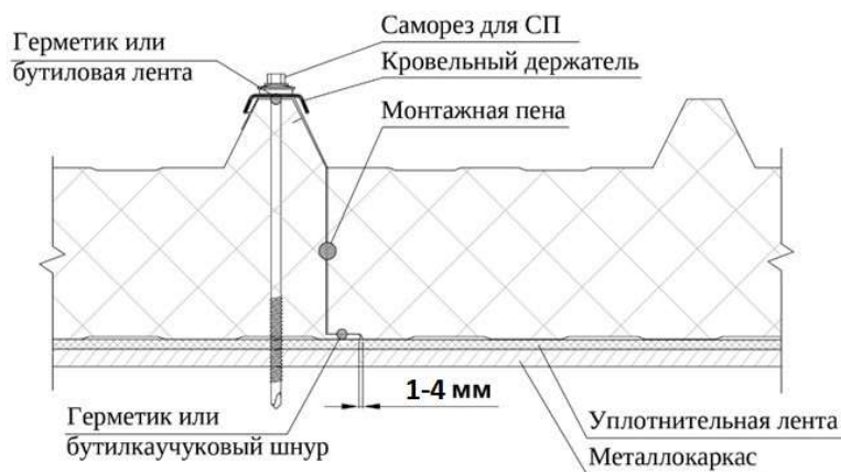
Рисунок 9. Замок кровельных панелей
